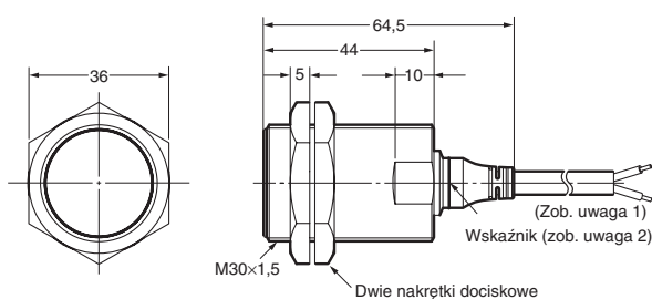
E2A-M30KS15-WP-□□/E2A-S30KS15-WP-□
