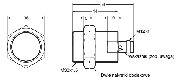
E2A-M30KS15-M1-□□/E2A-S30KS15-M1-□
