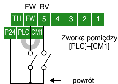
Sterowanie wspólnym plusem (nastawa fabryczna):
