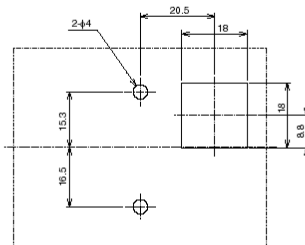
Otwór pod montaż panela
