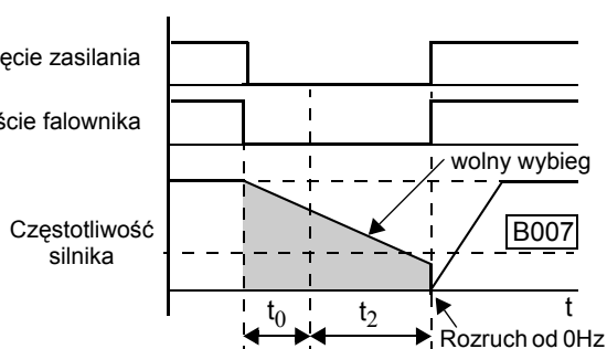
Przykład 4: Ponowny rozruch od 0Hz
