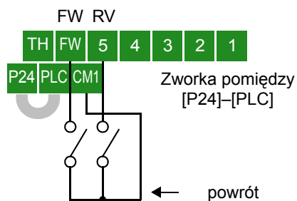
Sterowanie wspólnym minusem:
