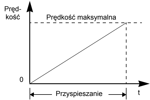
Nastawiony czas przyspieszania
