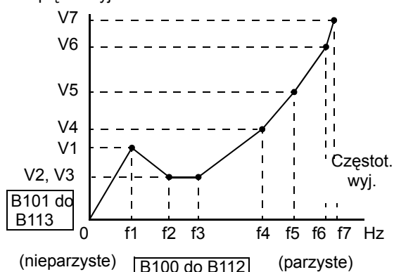
Napięcie wyjściowe
